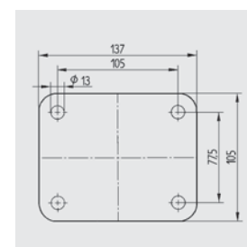
P67-137x105 Swivel castors
